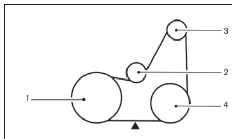
Κινητήρας K9K
