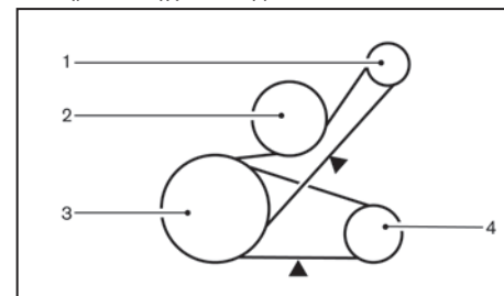
Κινητήρας BR10DE
