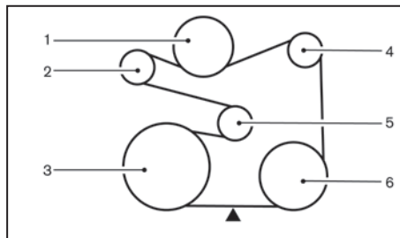
Κινητήρας HR09DET
