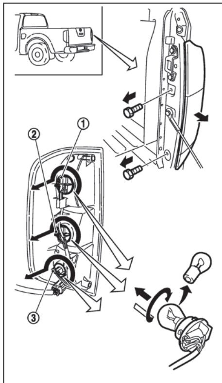
Συνδυασμός πίσω φώτων (φλας, στοπ και όπισθεν) (μοντέλα με κουτί καρότσας)
