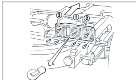
Συνδυασμός πίσω φώτων (φλας, στοπ και όπισθεν) (μοντέλα χωρίς κουτί καρότσας)
