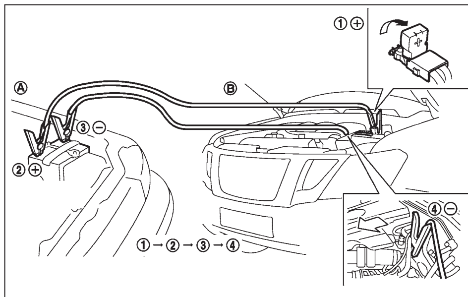
Μοντέλα με κινητήρα YD25DDTi
