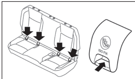
Θέσεις σημείων στήριξης ISOFIX
