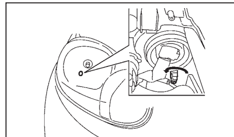
Εμπρός πλευρικό φως πορείας (παράδειγμα)
