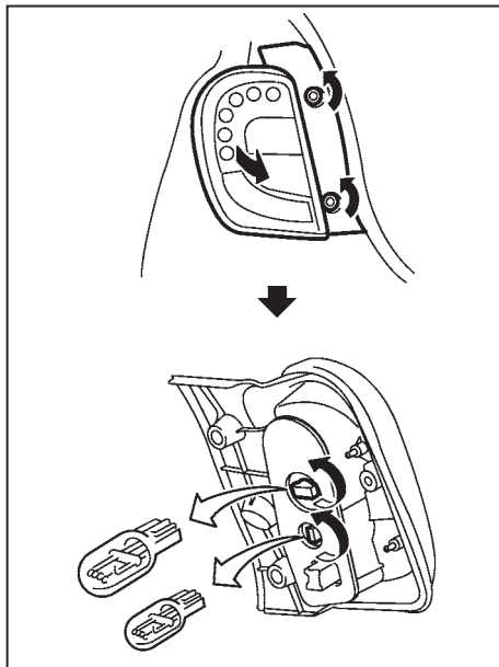
Συνδυασμός πίσω φώτων (Τύπος Β)
