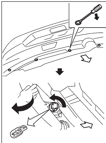
Πίσω φως ομίχλης
