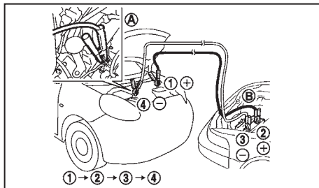
Μοντέλα με κινητήρα HR12DE
