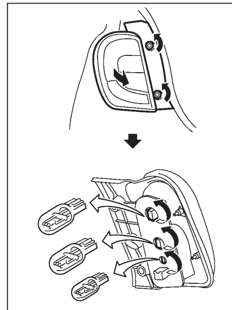
Συνδυασμός πίσω φώτων (Τύπος Α)
