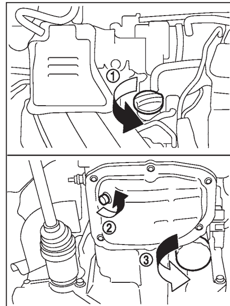
Μοντέλο κινητήρα HR12DE
