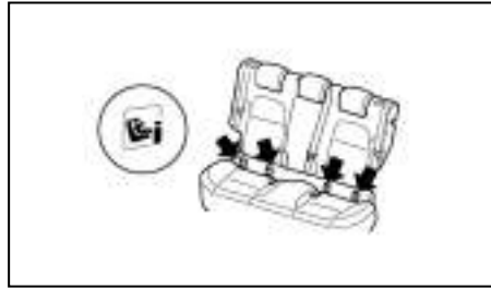
Θέσεις σημείων στερέωσης ISOFIX πίσω
