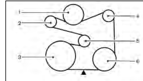
Κινητήρας HR09DET
