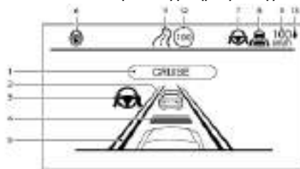
Μοντέλα με αναλογικό μετρητή και έγχρωμη οθόνη
