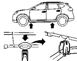
Σημεία στερέωσης του γρόλου
